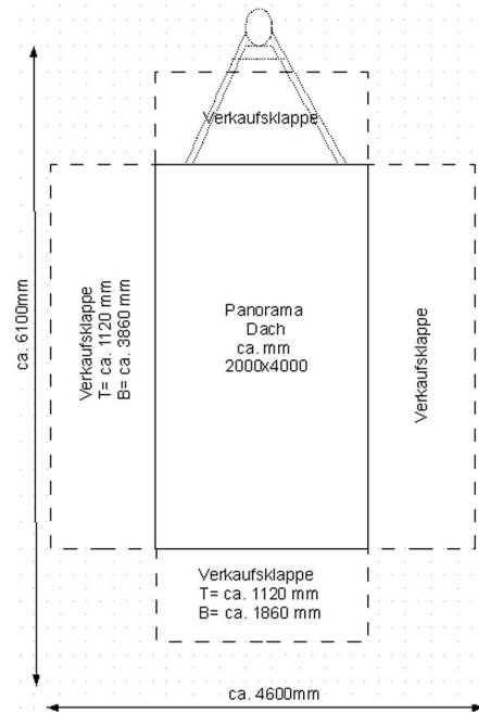
Abmessungen Draufsicht:
