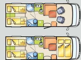
Grundrissbeispiel Tag | Nacht
